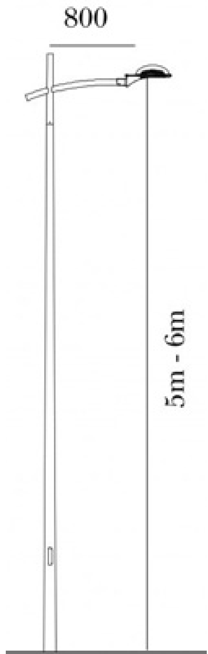
Pali Illuminazione Scala 1:50
